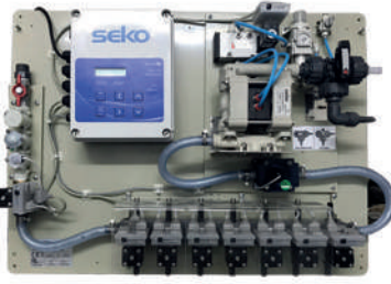
Çamaşır Makinesi Merkezi Sıvı Dozaj Sistemi
